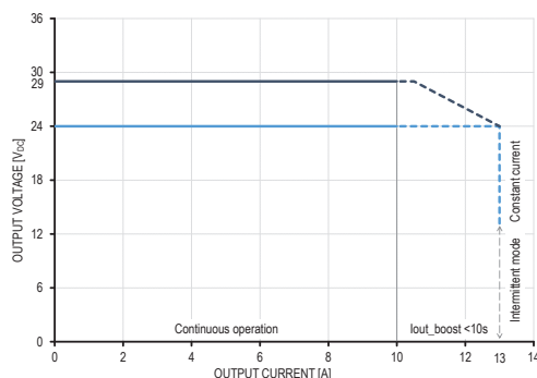
Fig. 4: Boost current capability up to 55°C amb
