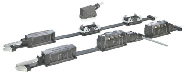
Abbildung 5: Beispiele von Anschlussmodulen mit Einspeisung über Rundleitung 400/480 V AC und 24 V DC.
