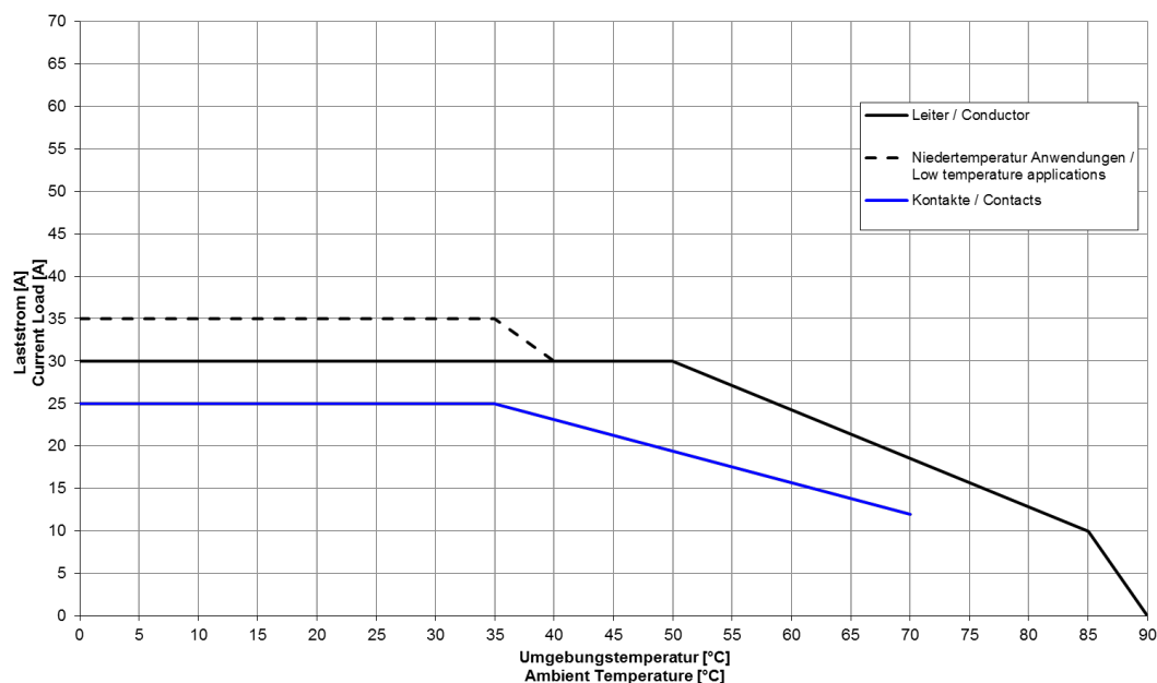
Diagramm 1: Maximal zulässige Strombelastung pro Leiter und Kontakt bei Laststrom auf L1, L2 und L3, für Flachleitung EVA 7G4 (00.709.0504.1) und Flachleitung XLPE (00.729.0504.1), gespeist über Stecker komplett FCS 4 7 ST SA SO0 (75.015.0151.0) und Flachleitungsabgang FCS 4 7 SI BU SW FM (99.800.4866.1).
