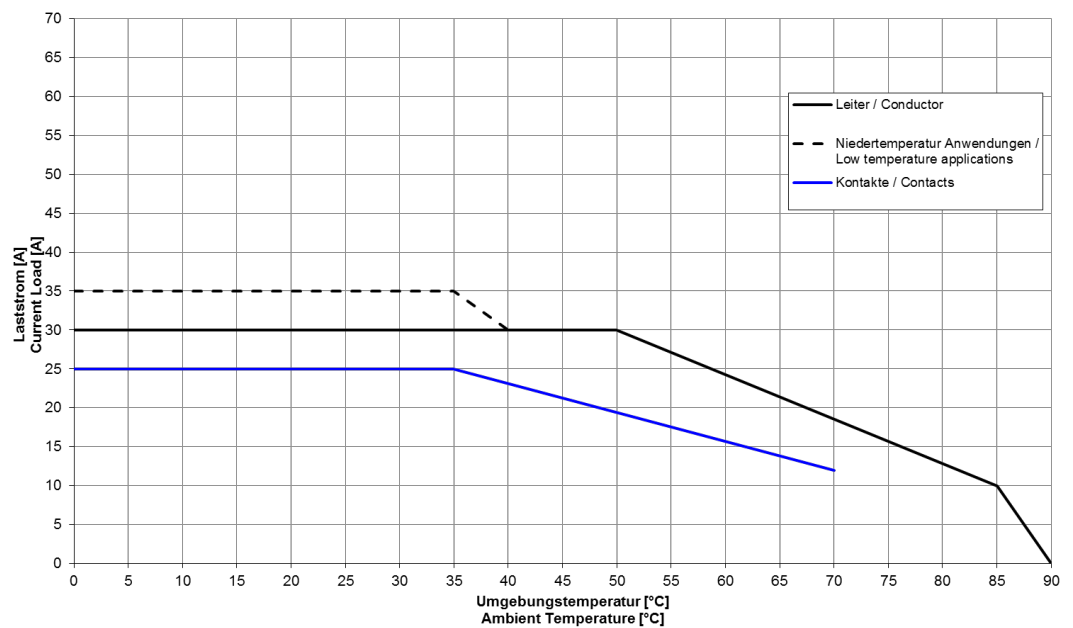
Diagramm 2: Maximal zulässige Strombelastung pro Leiter und Kontakt bei Laststrom auf L1, L2 und L3, für Flachleitung EVA 7G4 (00.709.0504.1) und Flachleitung XLPE (00.729.0504.1), gespeist über Stecker komplett FCS 4 7 ST SA SO0 (75.015.0151.0) und Flachleitungsabgang.
