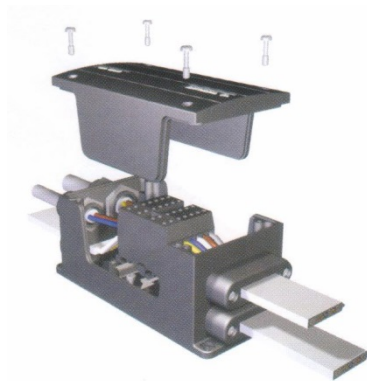
Abbildung 4: Verteilermodule mit Einspeisung über Rundleitung 400/480 V AC und 24 V DC, drei ausgehende Flachleitungen.
