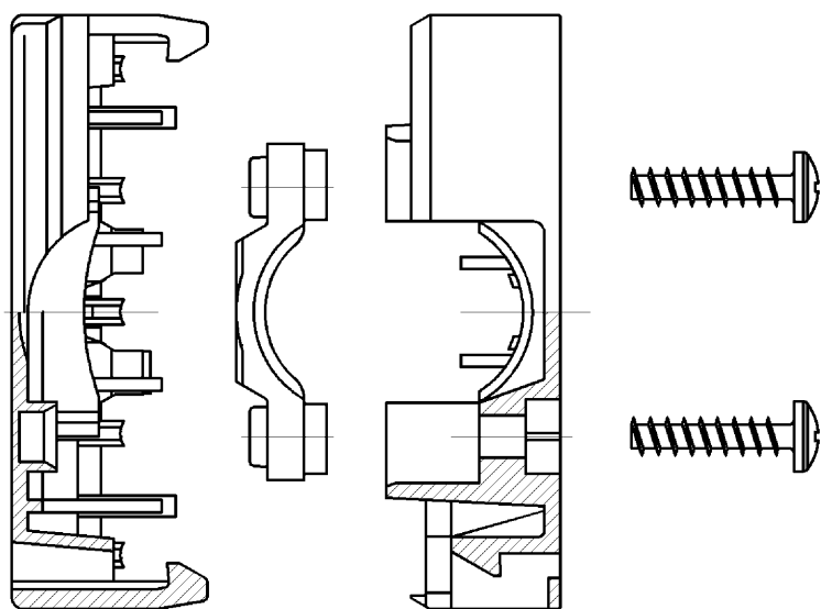
Teilschnitt B-B
